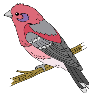
dziwonia
